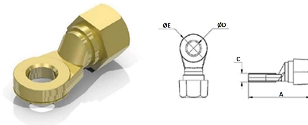
Figura 2 - Conector Lateral Reto
