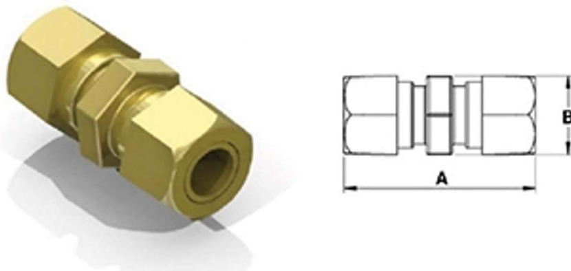
Figura 1 - Conector União Reto
